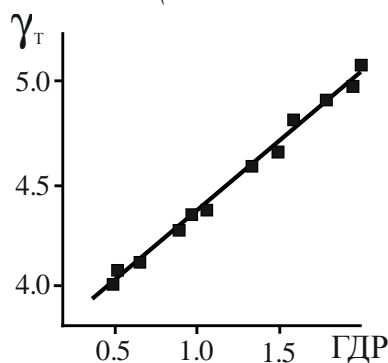
Рис. 3. Вплив рівня ЕМП ( ГДР = 50 \text{ В/м} , f=50\text{кГц} ) на \gamma_t захисту сталі 20 від малоциклової втоми в річковій воді (р. Десна)
