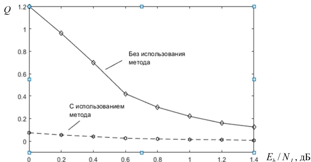
Рисунок 1 – Результаты моделирования характеристик передачи дополнительных бит для блока данных размером N = 6144
