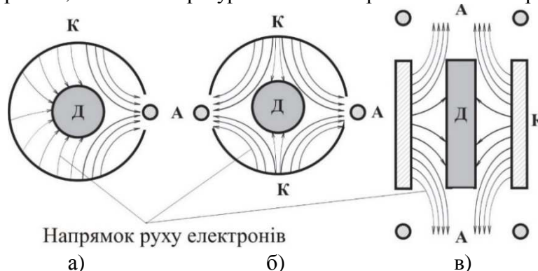
Рис. 1. Схема нагріву тліючим розрядом в порожнистому катоді: а) схема з одним каналом виходу електронів; б, в) схеми з двома каналами виходу електронів; А – анод; К – катод; Д – деталь.
