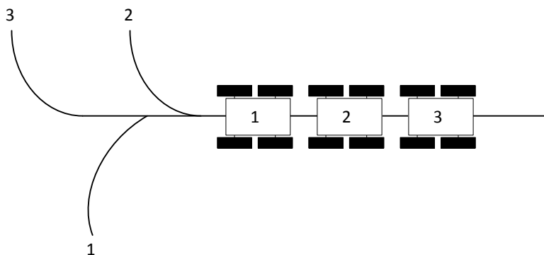
Obr. 1 Spomalenie materiálového toku v dôsledku spoločnej dráhy robotov
