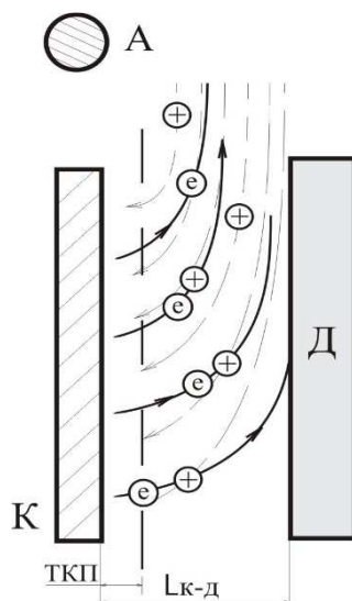
Рис. 2. Електричне поле тліючого розряду з порожнистим катодом: e – напрямок руху електронів; + – напрямок руху іонів; ТКП – темний катодний простір; L_{к-д} – відстань катод – деталь; А – анод; К – катод; Д- деталь.
