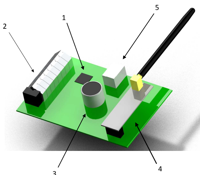
Obr. 4 Navrhnutý modul vysielača/prijímača, 1-mikrokontrolér, 2-pripojovacie svorky, 3-prijímač/vysielač, 4-anténa, 5-USB B konektor
