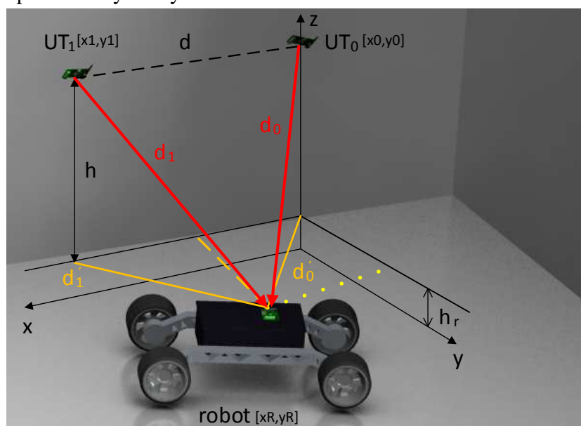
Obr. 3 Vzťah súradníc robota so súradnicami systému
