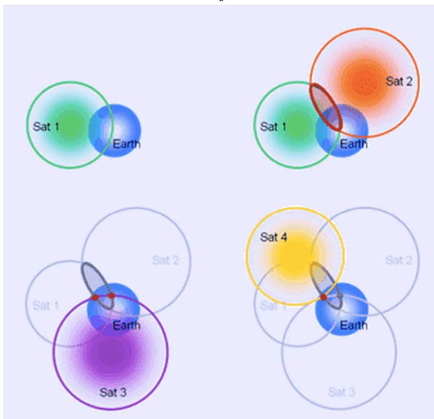
Obr. 2 Základný princíp trilaterácie použité na GPS [1]
