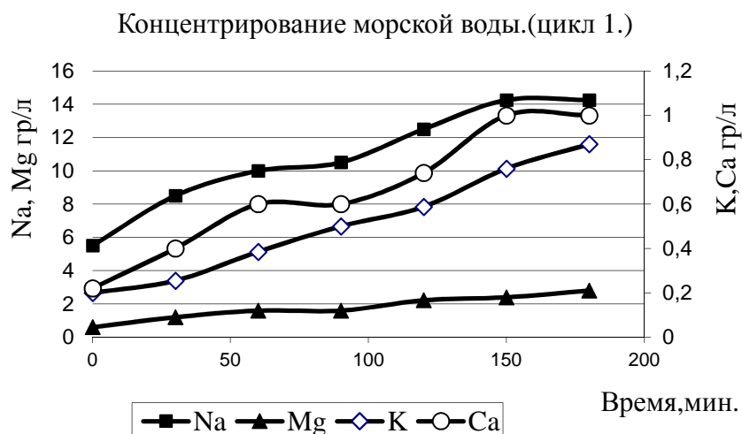
Рис. Концентрирование морской воды в процессе электродиализа
