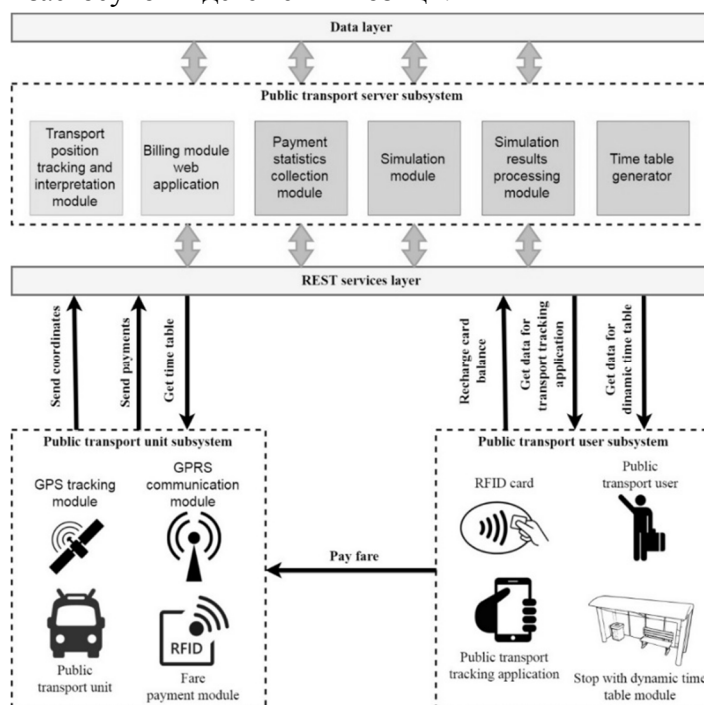
Рис. 1. Архітектура автоматизованої системи управління міським транспортом
