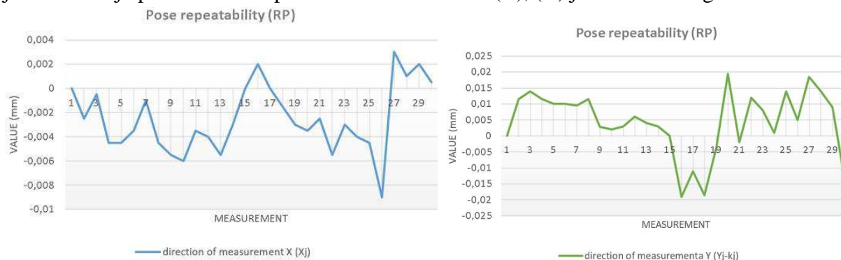
Obr. 3 Jednosmerná opakovateľnosť polohovania v osi X,Y / Pose repeatability in axis X,Y
