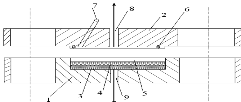
Рис. Мембранная ячейка:
