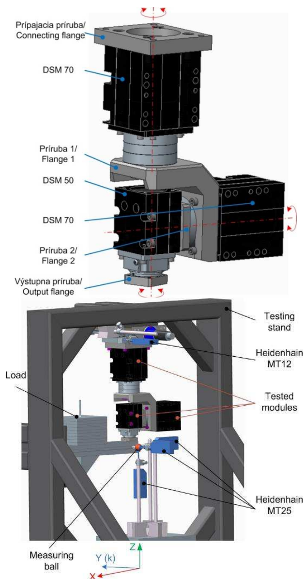
Obr. 1 Zostava zápästia v stende / Wrist assembly in stand
