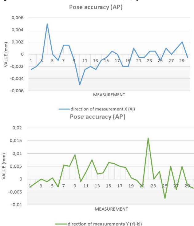
Obr. 2 Jednosmerná presnosť polohovania v osi X,Y / Pose accuracy in axis X,Y
