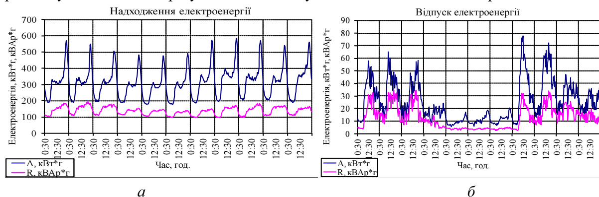
Рис. 3. Приклад виміряних значень протягом одинадцяти днів: а – надходження електроенергії з головної ділянки фідера; б – відпуск електроенергії по ТП-543
