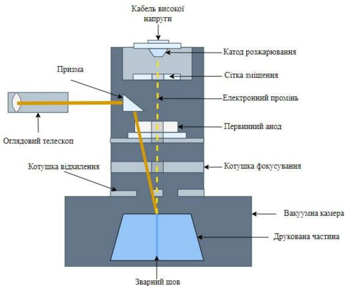
Рисунок 3.13 – Принцип роботи принтеру за технологією EBМ
