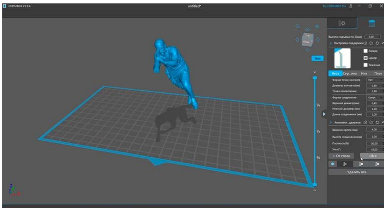
Рисунок 4.8 – Интерфейс ChiTuBox
