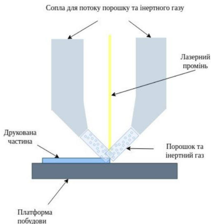
Рисунок 3.2 – Принцип роботи принтеру за технологією LENS Building
