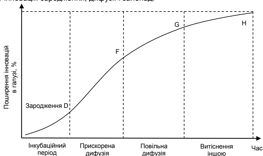
Рис. 4. Класична крива поширення інновацій: D, F, G, H – точки зміни стану процесу дифузії інновацій
