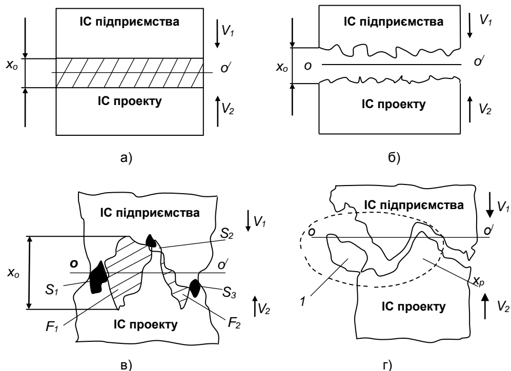
Рис. 1. Схема об'єднання двох інформаційних систем: 1 – локальний енергетичний потенціал; oo' – стан рівноваги
