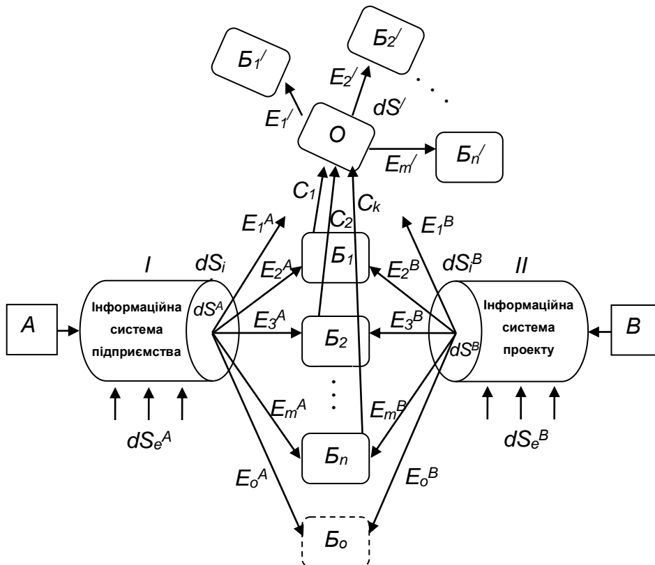
Рис. 2. Синергетична модель об'єднання двох інформаційних систем:
