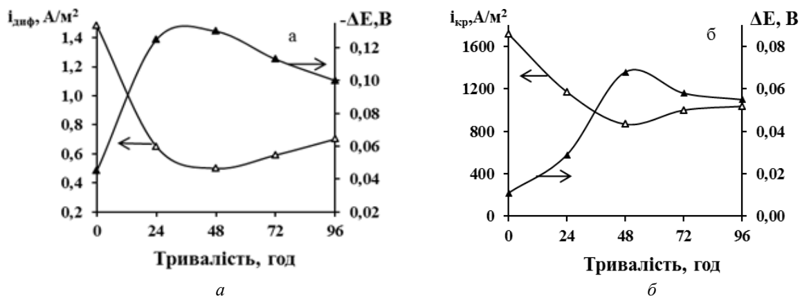
Рис. 2. Залежність густини струму для катодної області ( i_k ) (а) та для анодної області (при E = -0,3В ) (а) (б) і електродної поляризації ( \Delta E ) на Ст3 у розчині 1 н Na_2SO_4 залежно від тривалості оброблення сталі в паровій фазі рослинних екстрактів
