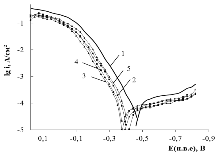
Рис. 1. Анодні (1–5) і катодні поляризаційні криві на сталі Ст3 у розчині 1 н \text{Na}_2\text{SO}_4 без (1) і з плівкою, отриманою після формування 24, 48, 72, 96 годин (2–5) у паровій фазі екстракту шишок хмелю
